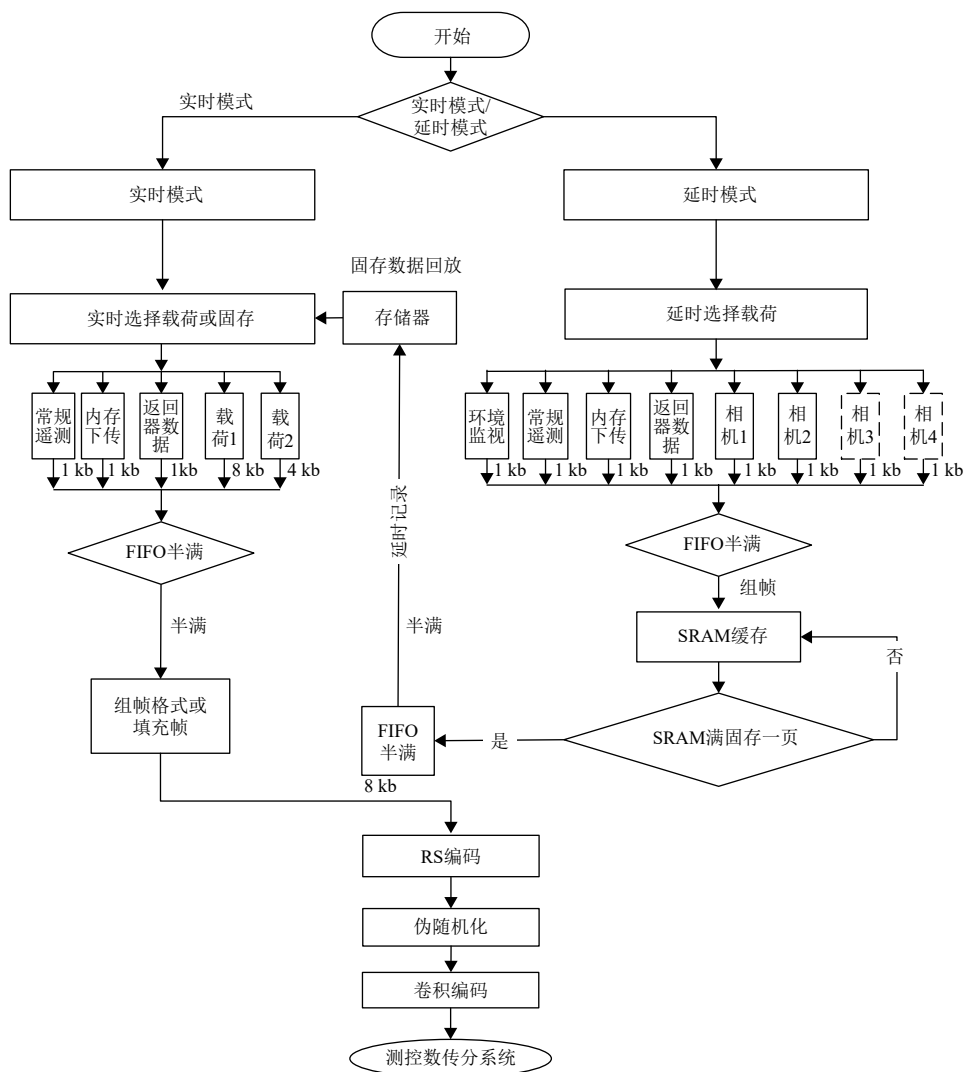
图4 数据存储信息流程图
