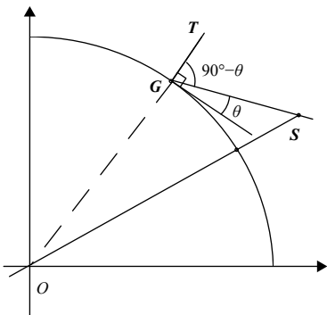
图2 测站与返回器位置关系
