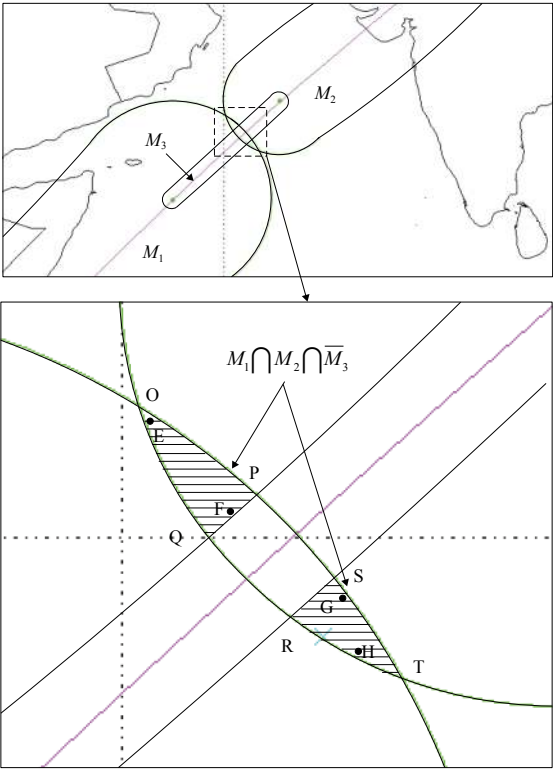
图7 海上测量船布设区域 Fig. 7 The space tracking ship visible region for reentry module
