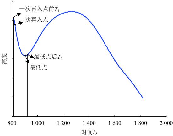
图 6 返回器一次再入及最低点高度变化曲线 Fig. 6 The altitude of reentry module
