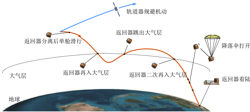
图1 “嫦娥五号”任务再入返回过程示意图 [14]
