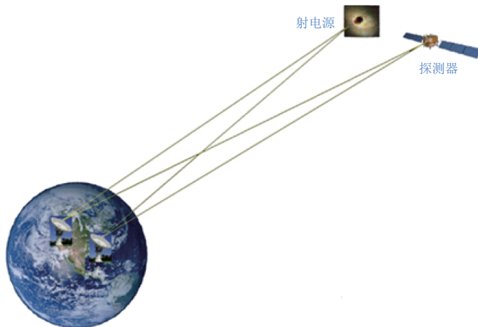
图2 差分干涉测量原理图
