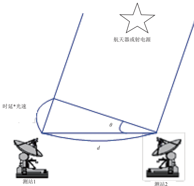
图1 干涉测量原理图
