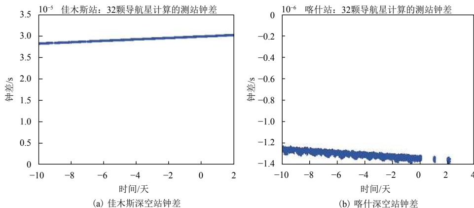
图3 佳木斯及喀什深空站5月21日至6月2日钟差
