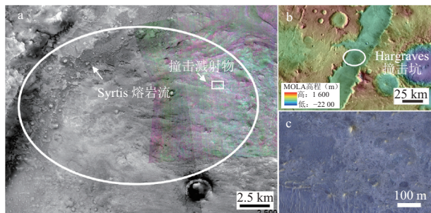
注：a为Nili Fossae（中心位置约21.0°N，74.5°E）的地貌。底图为火星专用小型侦查成像光谱仪的影像（红：D2300，绿：LCPINDEX2，蓝：BD1900）叠加在背景相机影像上。不同的颜色表明了不同的成分：红色表示粘土矿物，绿色表示低钙辉石。白色椭圆为建议的着陆椭圆，大小为25 km × 20 km。箭头分别指示Syrtis的熔岩流与撞击溅射物；b为Nili Fossae的地形地貌图，为MOLA数字高程图叠加在THEMIS昼间热红外图像；c为Hargraves撞击溅射物，HiRISE影像。
