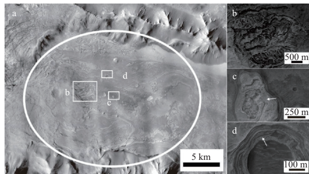
注：a为SW Melas的CTX影像（中心位置约为9.8°S，283.6°E），白色椭圆为建议的着陆椭圆，大小为25 km × 20 km；b为水下三角洲地貌；c为水合硅土；d为撞击坑坑壁出露的层状结构。b、c、d为HiRISE影像。
