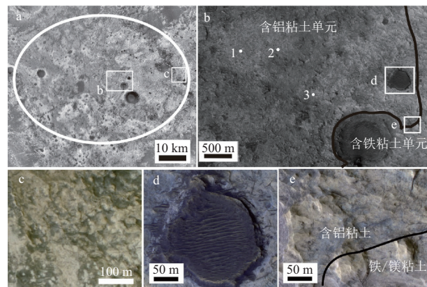
注: a为Mawrth Vallis (中心坐标约 22.3^{\circ}\text{N} , 343.5^{\circ}\text{E} ), CTX拼接图像。白色椭圆为建议的着陆椭圆, 大小为 25\text{ km} \times 20\text{ km} ; b出露了大量与水环境相关的矿物。点1探测到了高岭石/明矾石。点2探测到了黄钾铁矾。点3探测到了Al蒙脱石; c为斑点状构造; d为黑色盖层残余, 覆盖在黏土矿物之上, 可能为黏土矿物的形成时间提供限制; e为Fe黏土单元和Al黏土单元, 它们有明显的边界。b、c、d、e为高分辨率影像科学仪器(High Resolution Imaging Science Experiment, HiRISE)影像。
