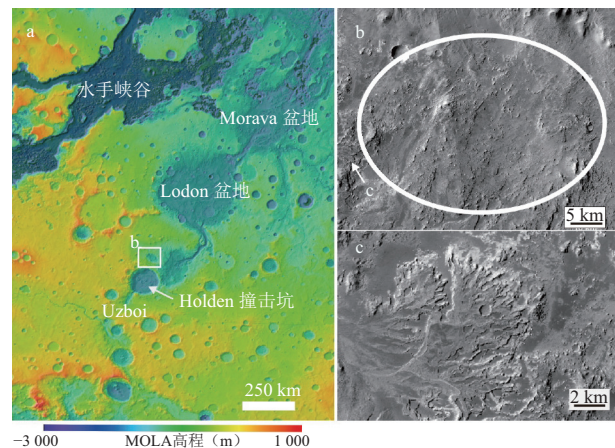
注: a为Uzboi-Ladon-Morava (ULM) 河谷盆地系统, 火星轨道高程数据叠加在热发射影像系统昼间热红外图像上; b为Eberwalde撞击坑(中心坐标约 24.0^{\circ}\text{S} , 327.0^{\circ}\text{E} ), 白色椭圆为建议的着陆椭圆, 大小为 25\text{ km} \times 20\text{ km} , 白色箭头处为Eberwalde撞击坑的三角洲所在的位置。为背景相机拼接图像; c为Eberwalde撞击坑内西部的三角洲, 可能保存了古老生物痕迹。
