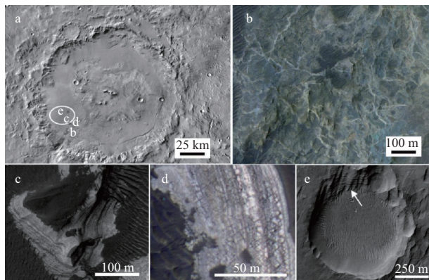
注：a为Holden撞击坑（中心坐标约26.4°S，325.1°E）的CTX影像。白色椭圆为建议的着陆椭圆，大小为25 km × 20 km。b、c、d、e来自HiRISE影像。b为Holden撞击坑里的撞击角砾岩；c为着陆椭圆内的一处含粘土矿物的浅色物质的露头，是寻找古老生命痕迹的理想地点；d浅色物质上可见有些多边形裂缝；e显示撞击坑坑壁的地层（白色箭头）出露良好。
