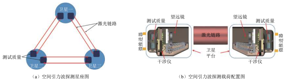
图2 空间引力波探测星座图和空间引力波探测载荷配置图
