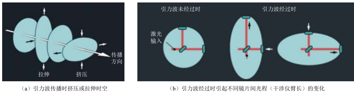
图1 引力波传播时挤压或拉伸时空和引力波经过时引起不同镜片间光程（干涉仪臂长）的变化
