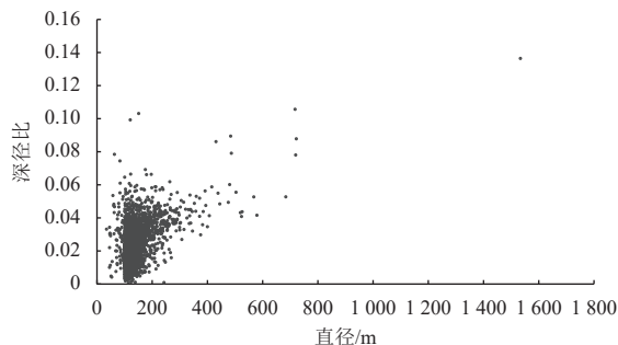
图8 典型区所有撞击坑的直径与深径比关系图
