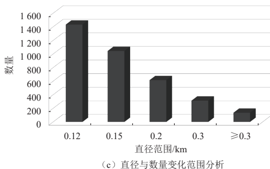
图3 研究区撞击坑分布情况、完整性分析及直径与数量变化范围(底图为5 m分辨率的CTX DOM影像)
