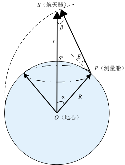
图4 测量船几何可见示意图
