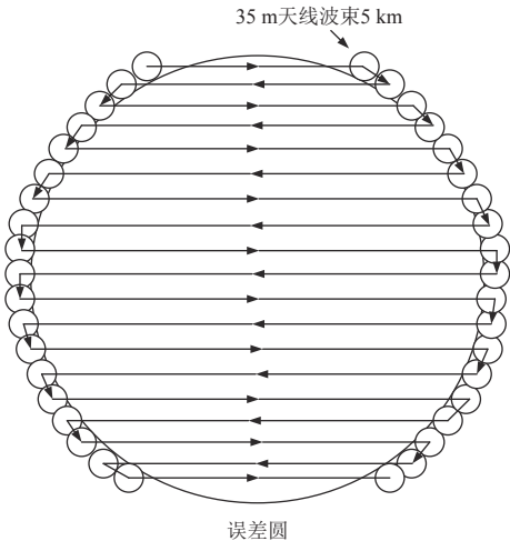
图 9 阿根廷深空站快速扫描捕获示意图 Fig. 9 Fast sweep capture of Argentina deepspace station
