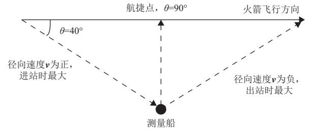
图3 测量船多普勒示意图 Fig. 3 Doppler of TT&C ship
