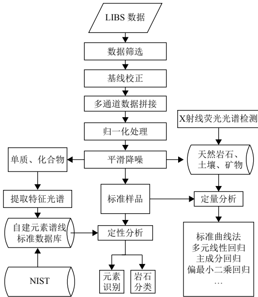
图6 LIBS数据分析流程图
