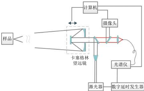
图1 远程LIBS分析系统框图
