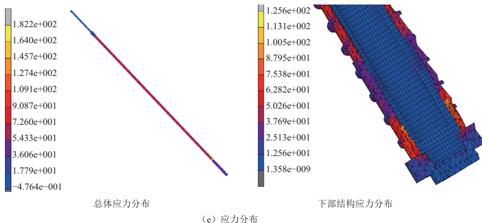
图6 钻具工作状态(最终状态)下的位移、温度和应力分布
