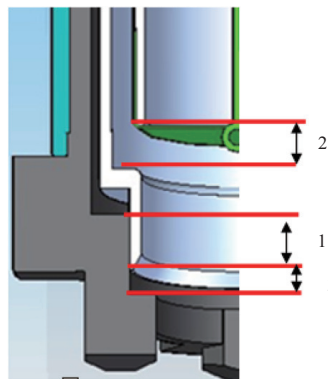
图4 低温、高温存储下钻头部位配合部位序号 Fig. 4 The assembly parts' serial number of drilling bit
