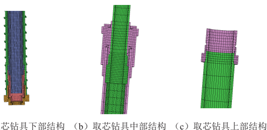
图1 取芯钻具热力耦合计算模型
